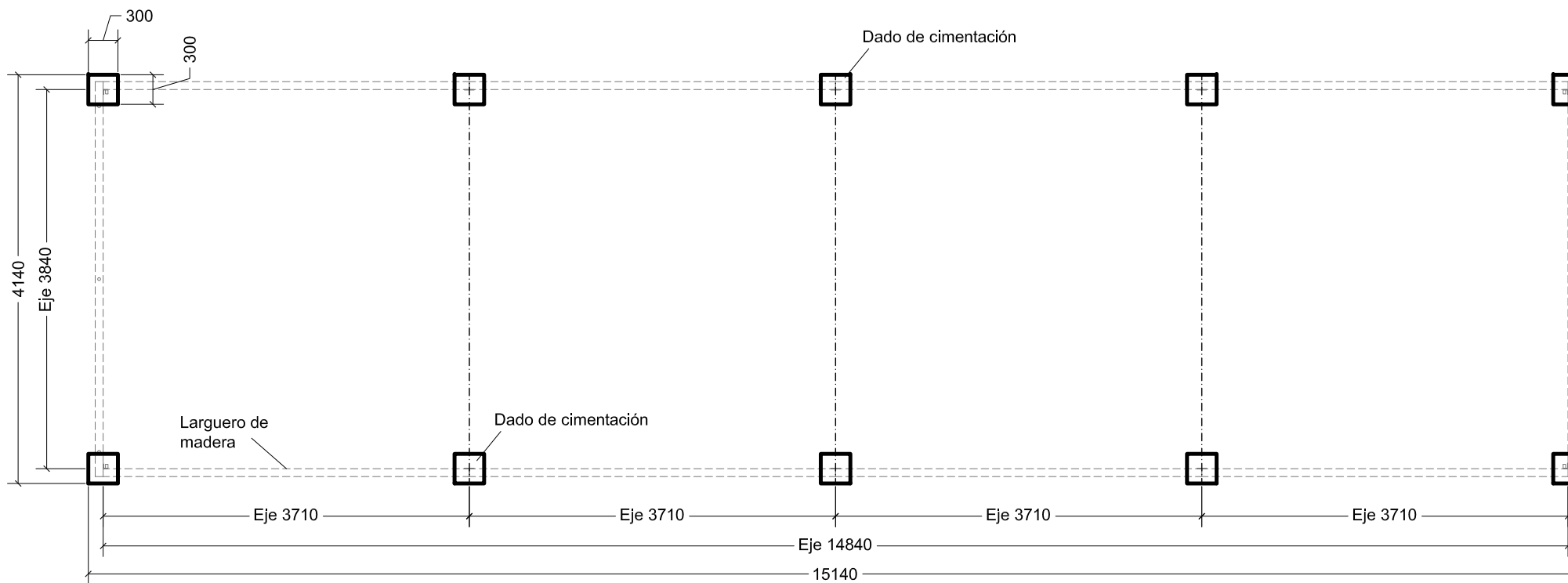
Planta de Cimentación
